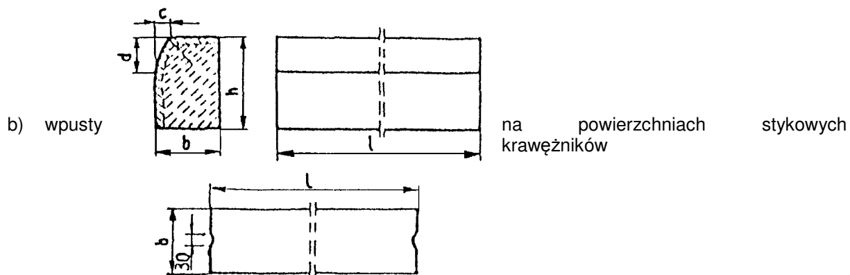
Rys. 1. Wymiarowanie krawężników
